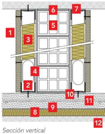
Sección vertical
