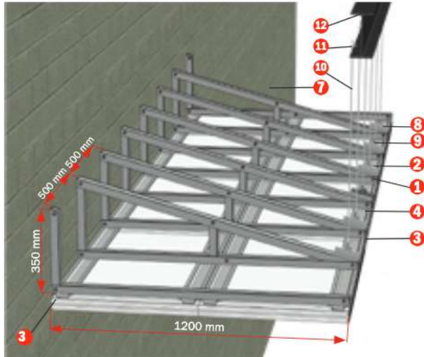
Sistema de montaje de la franja horizontal
