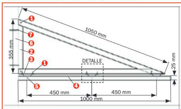
Sistema de montaje de la franja horizontal
