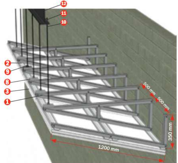
Sistema de montaje de la franja inclinada
