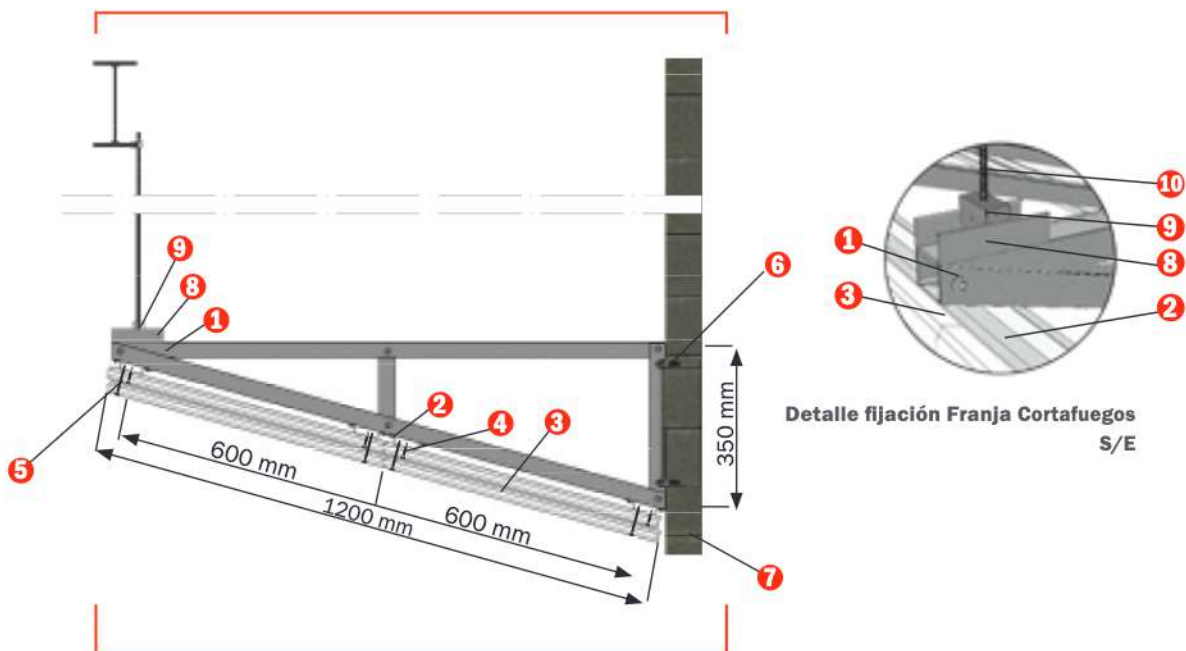
Sistema de montaje de la franja inclinada
