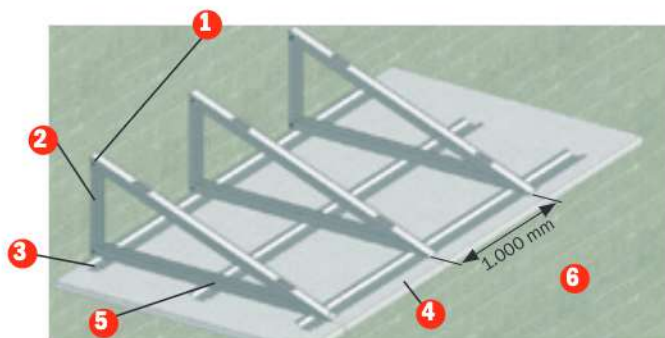
Sistema de montaje de la franja horizontal
