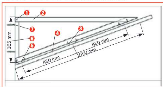
Sistema de montaje de la franja inclinada
