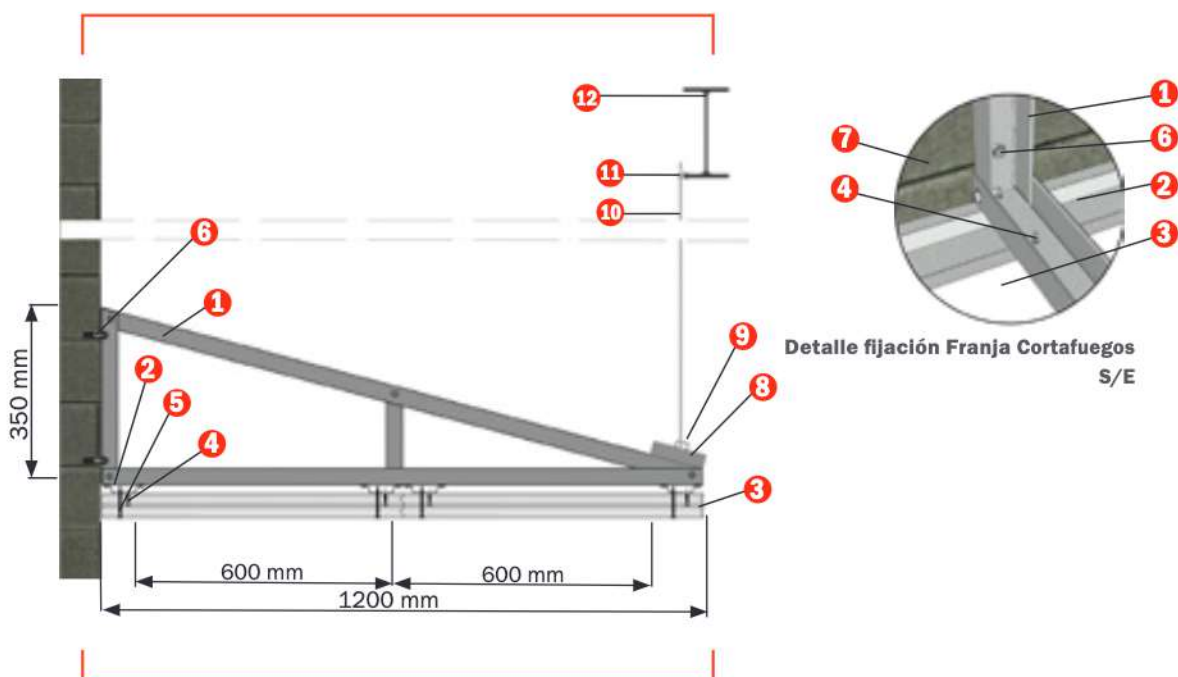
Sistema de montaje de la franja horizontal
