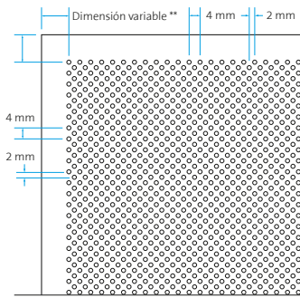
Perforación Ø 1,5 mm Área perforada ~ 22%
