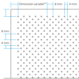
Perforación Ø 1,5 mm Área perforada ~ 5,5%
