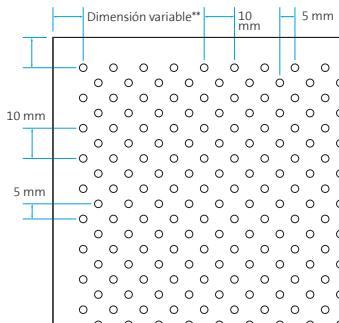
Perforación Ø 2,5 mm Área perforada ~ 10%
