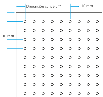
Perforación Ø 2,5 mm Área perforada ~ 5%
