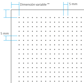
Perforación ultra-micro Ø 0,7 mm Área perforada ~ 1,5%
