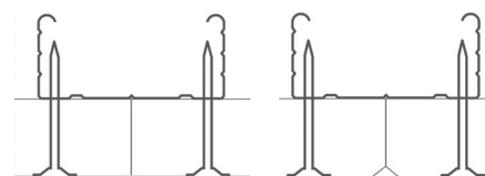
Perfil Oculto Atornillada K0
