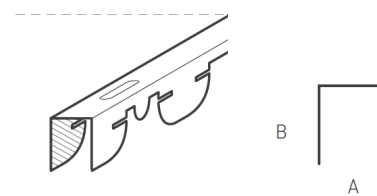
Rastrel para techo
